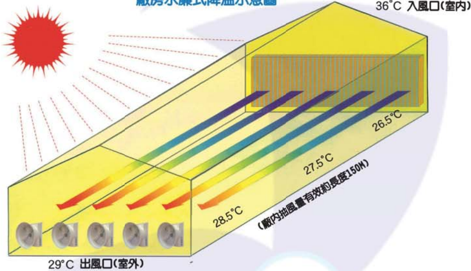
廠房水簾式降溫示意圖
